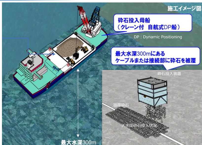
1. ①大水深碎石投入のイメージ 出典：古河電気工業株式会社 (本事業で洋上接続部などへの防護工法を開発予定)
