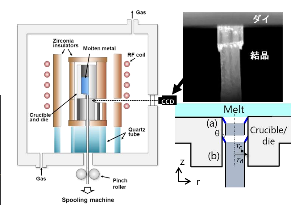
Dewetting μ-PD法
