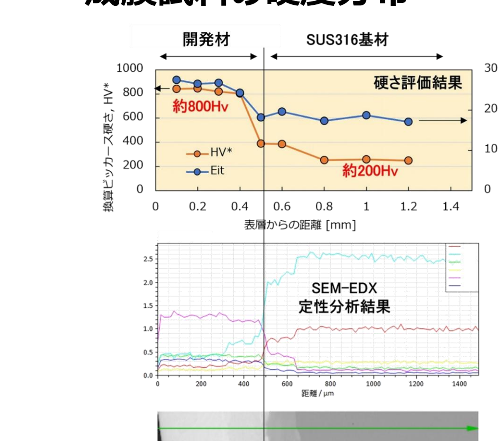
成膜部材の硬度分布と試験後の状態
