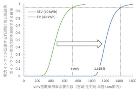
図2. レジリエンス; 太陽電池搭載車 (SEV) とEVの必要台数のシミュレーション結果例
