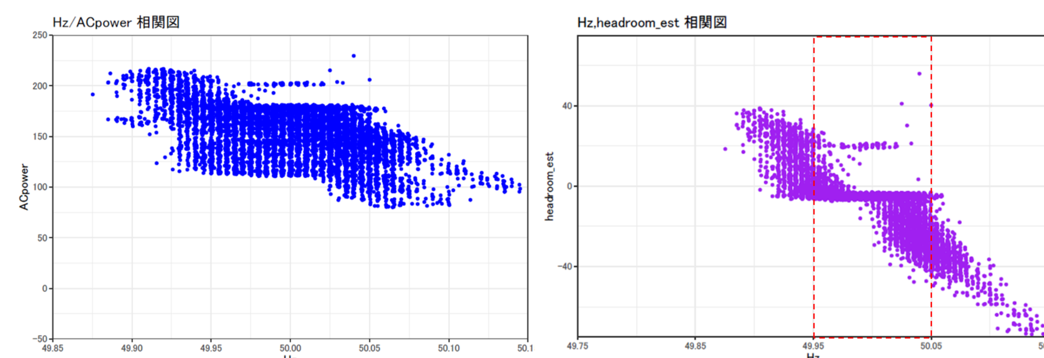
Δ制御：周波数とAC出力の関係（13:00～13:59）
