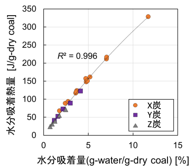
図 高感度TG-DSC
