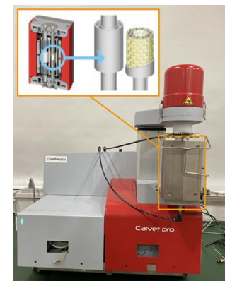
図 高感度TG-DSC
