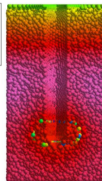
石炭充填層(R70装置) 温度分布の予測
