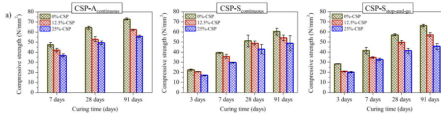
図1 製造方法が異なるCSPの形態とモルタルの強度
